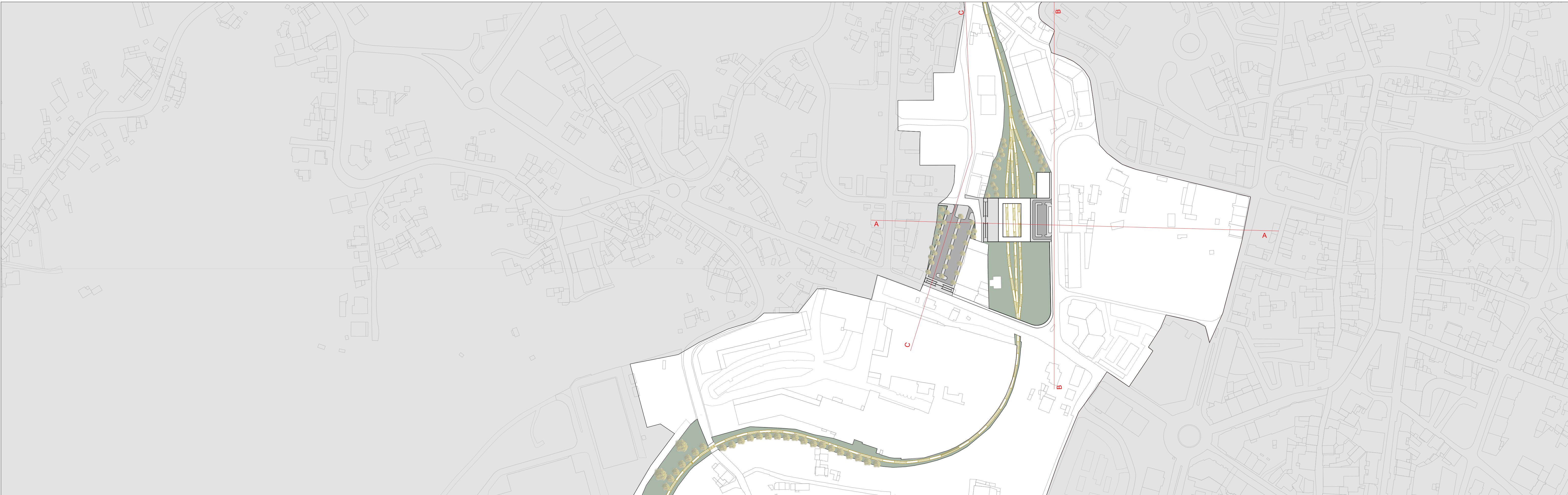
PLANTA ZONA DE INTERVENÇÃO PRIORITÁRIA 02 - ESTAÇÃO CENTRAL DE OLIVEIRA DE AZEIS - ESC. 1/2000
